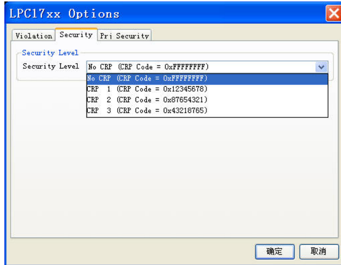
图 3.6 配置 LPC1766 的加密级别
