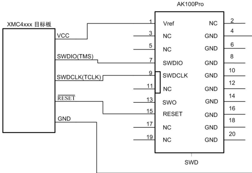
图 3.4 XMC4500-F100F1024 编程接口引脚定义
