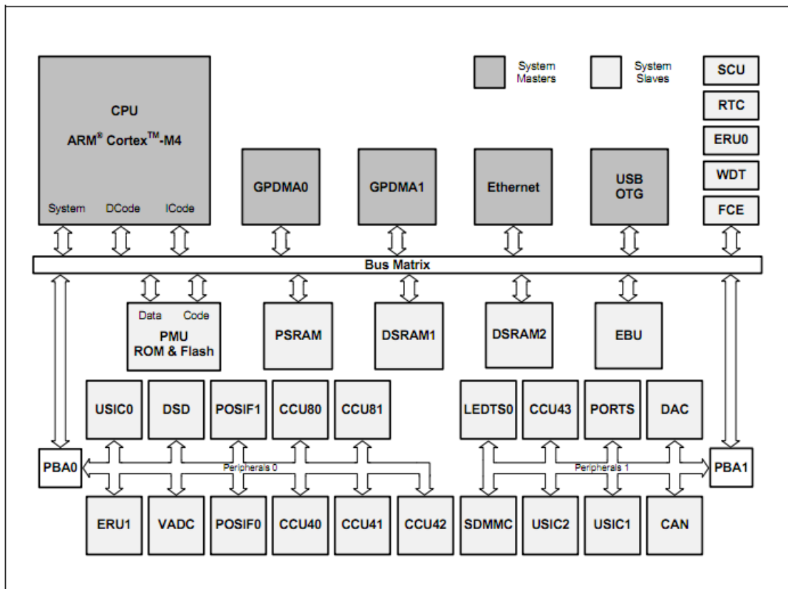
图 1.1 XMC1100-T038F-0064AA 内部结构框图
