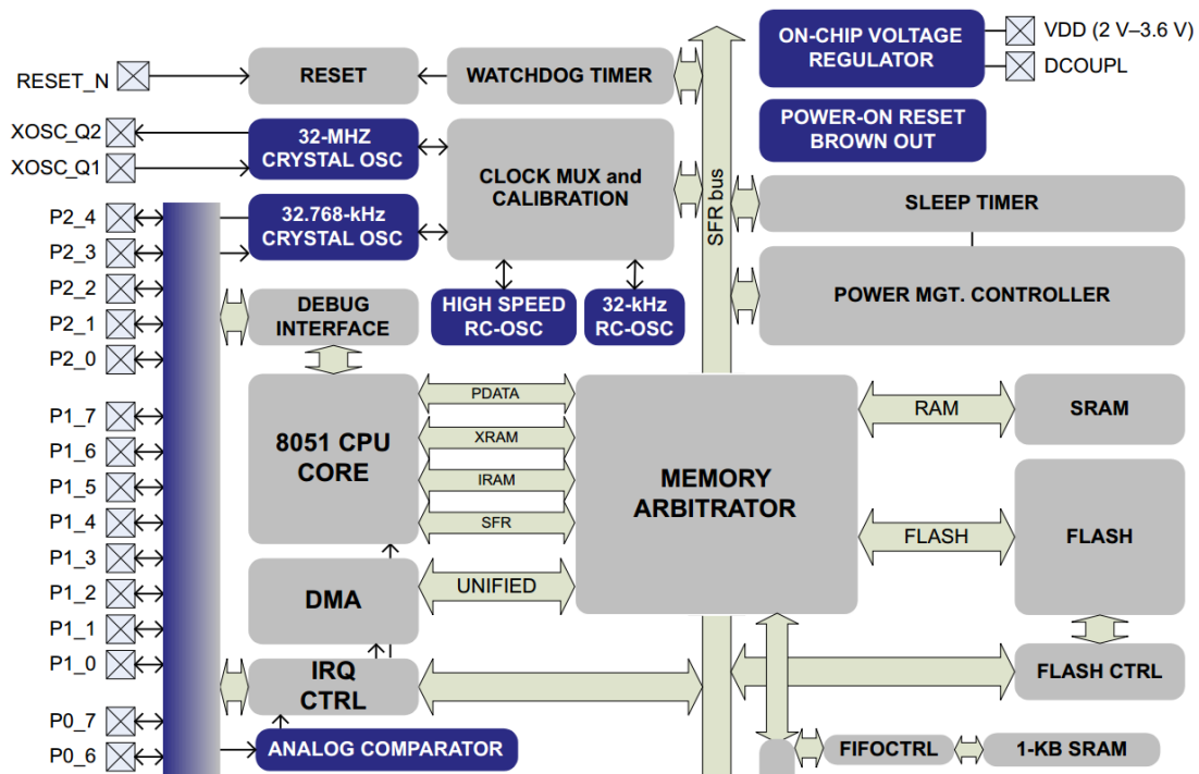
图 1.1 CC253x 部分内部框图
