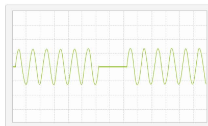
线路编程 (Sim) 仿真电压突降输出
