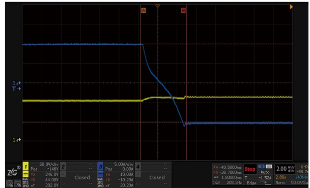
源载动态切换响应图
